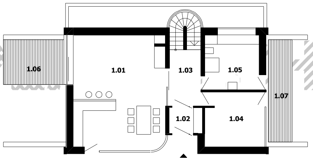
PŮDORYS 1.NP
